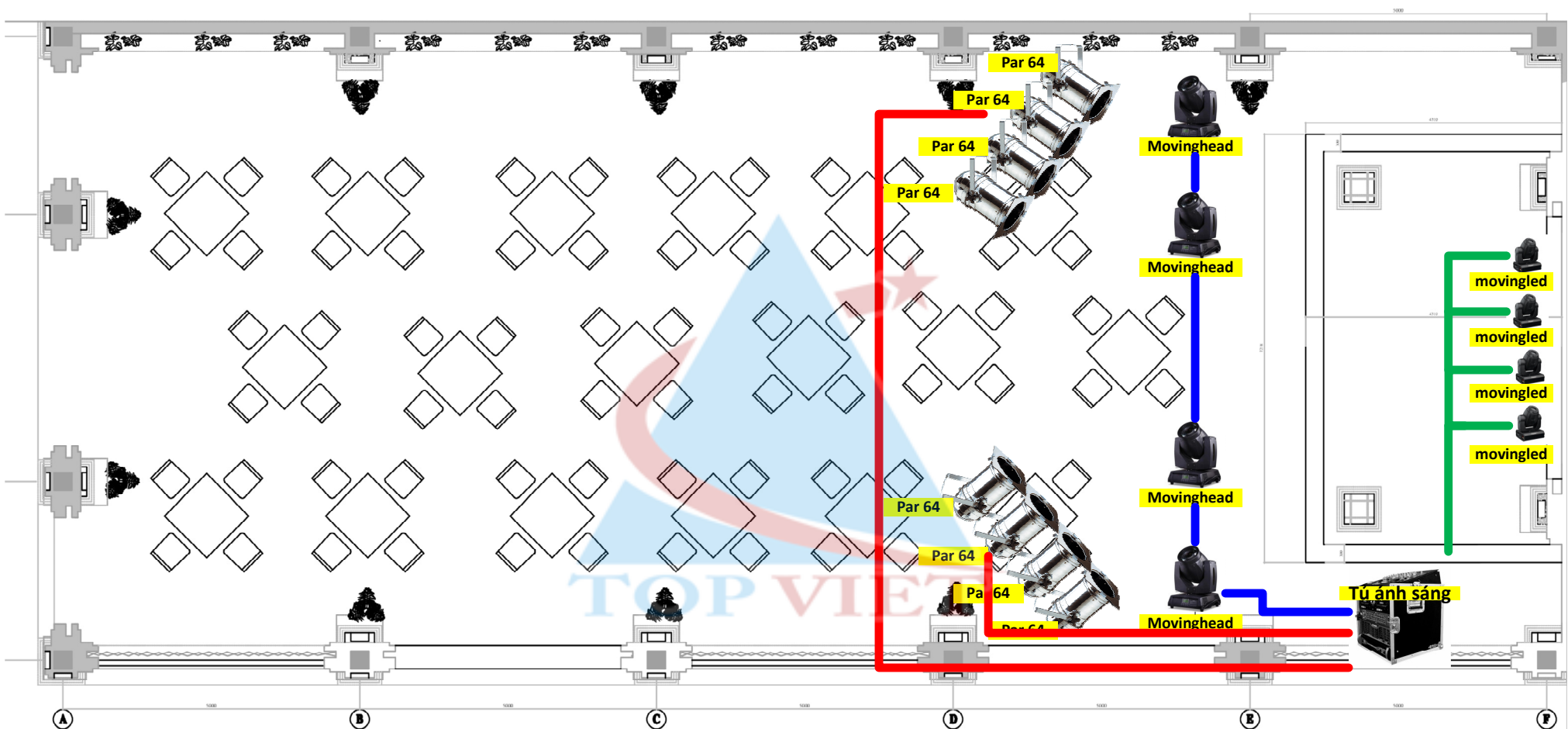
SƠ ĐỒ BỐ TRÍ HỆ THỐNG ÁNH SÁNG HỘI TRƯỜNG
