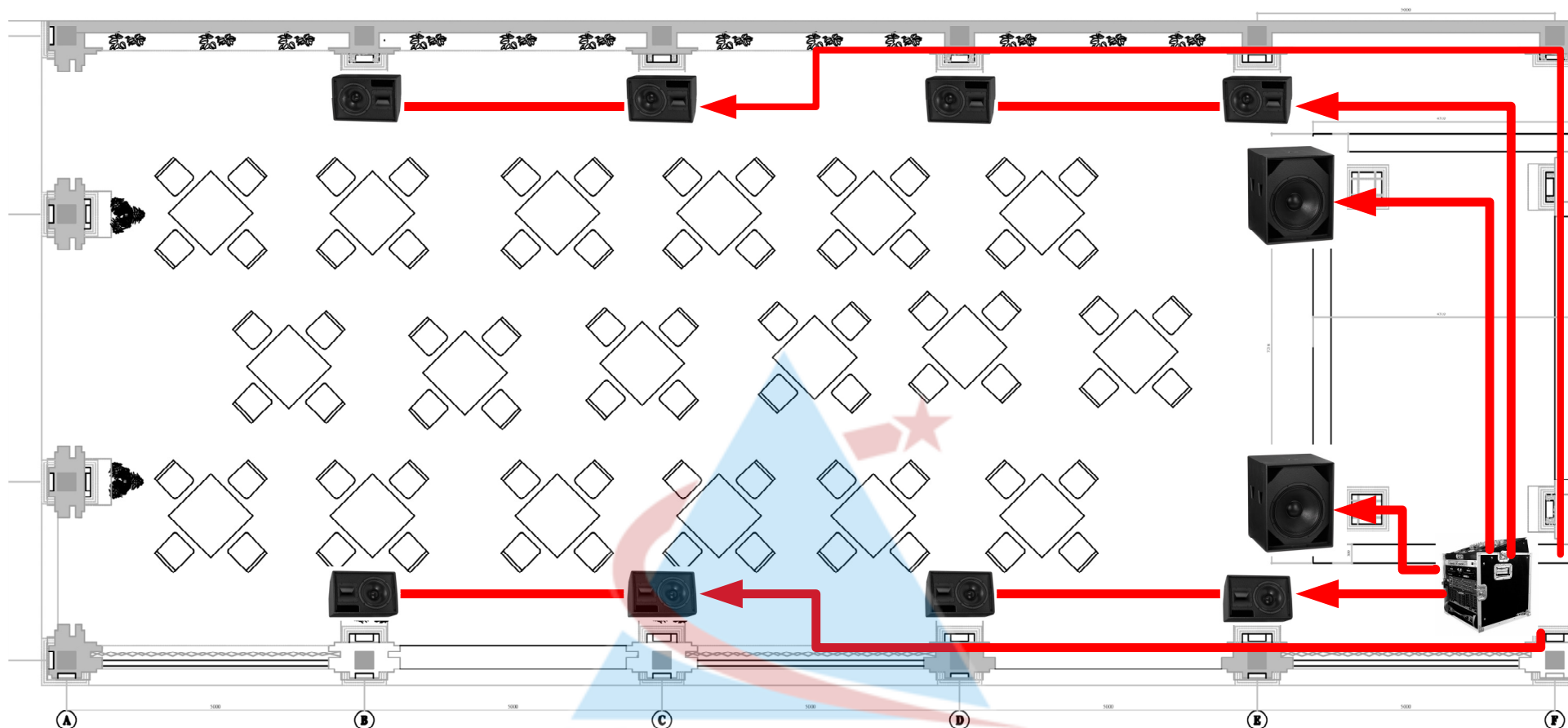
SƠ ĐỒ BỐ TRÍ HỆ THỐNG ÂM THANH HỘI TRƯỜNG
